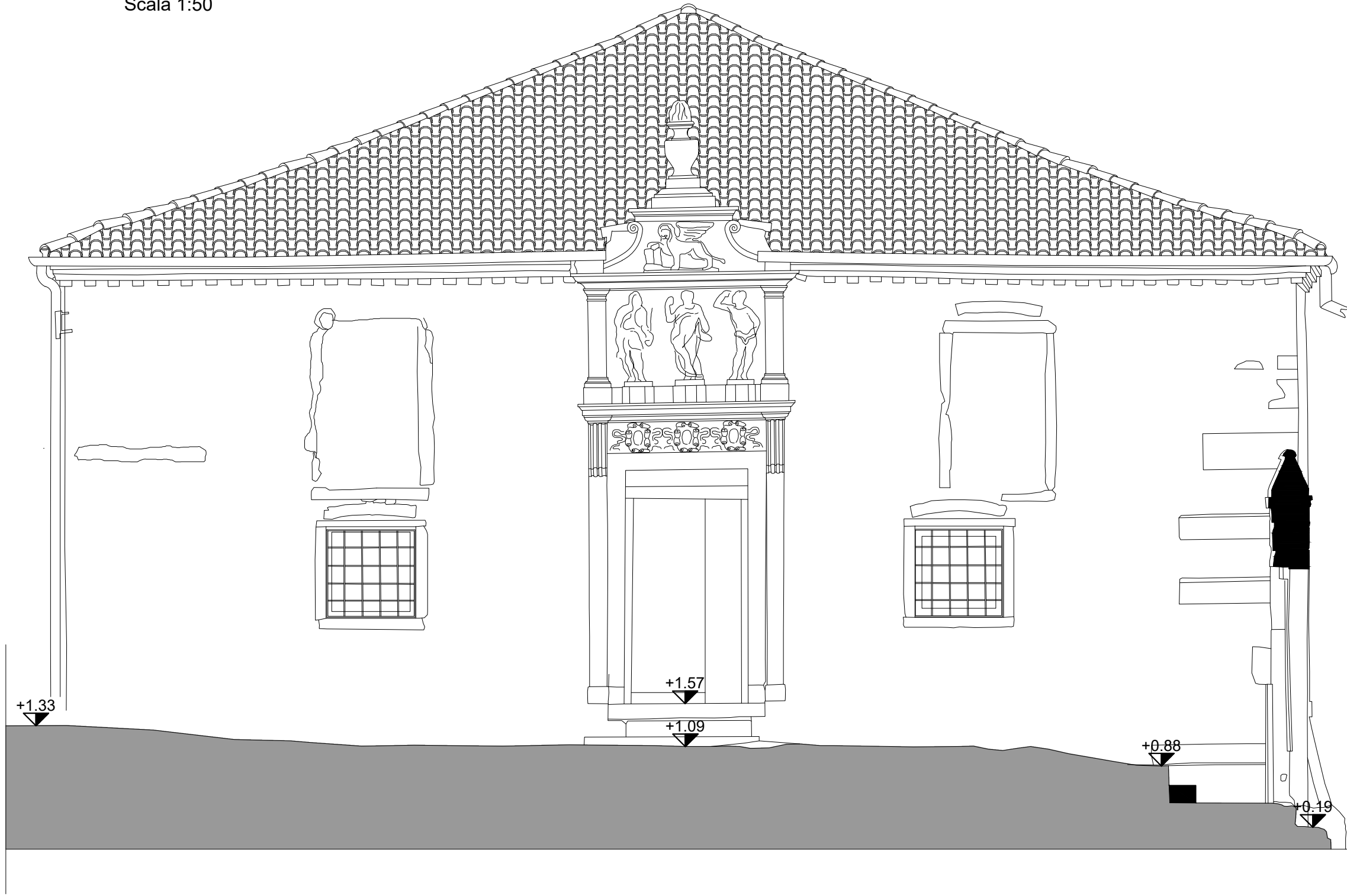
Prospetto Ovest Scala 1:50
