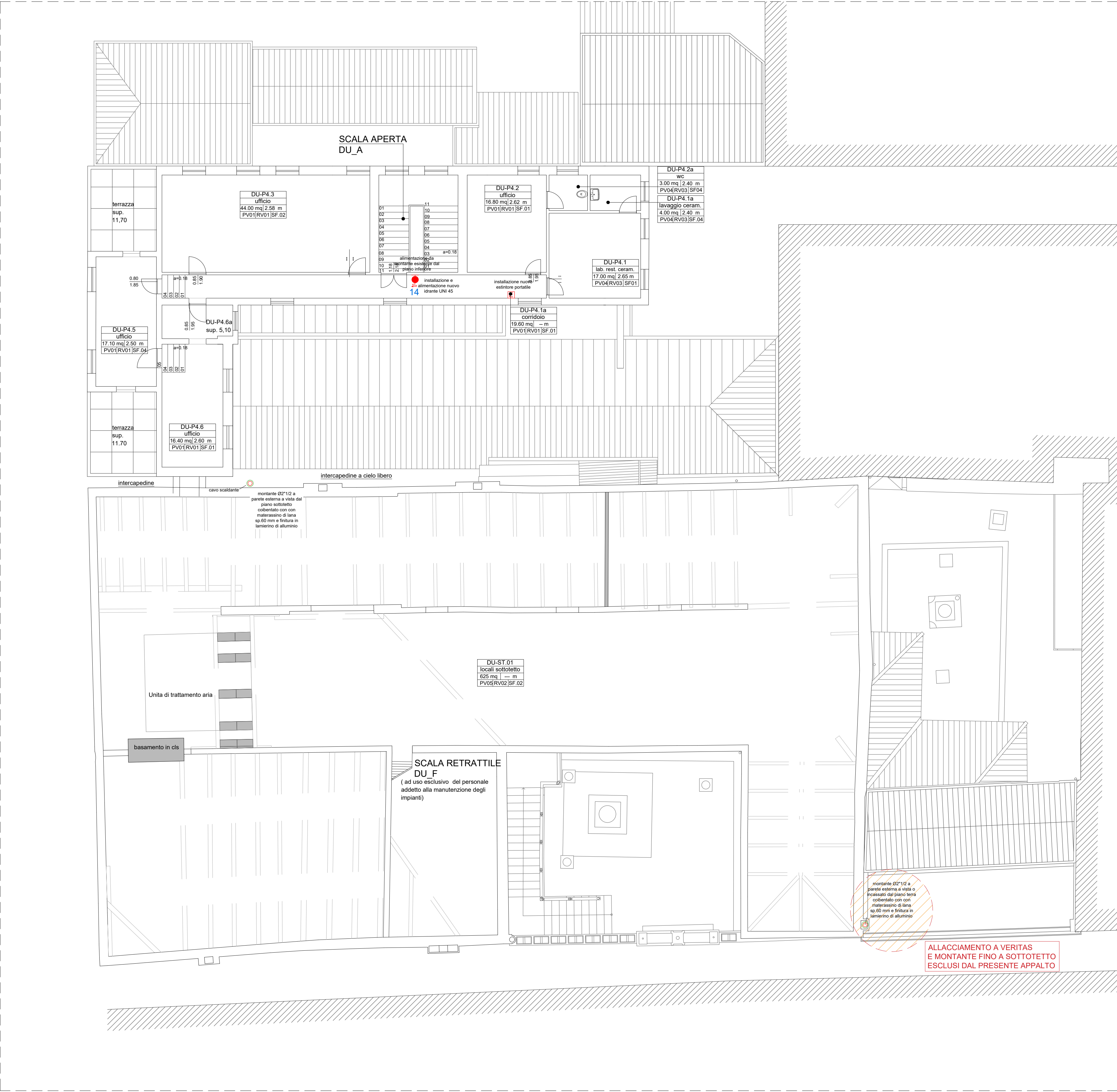
Palazzo Duodo - Pianta Piano Quarto Ca' D'Oro - Pianta Piano Secondo Impianto Antincendio Scala 1:100
